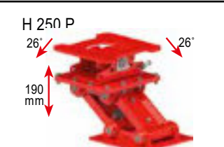
H 250 P Höhenausgleich H 250 P / 190 mm Ausgleich ↑↓ mit Pendelausgleich (Art.-Nr. 267.95.456) 1.790 €
