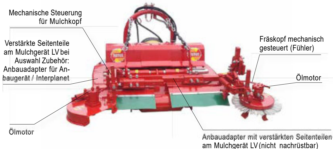
Mechanische Steuerung für Mulchkopf
