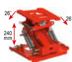
Höhenausgleich H 240 P / Parallelogramm 240 mm, Pendel links/rechts 26° (max. Gewicht Mulchkopf 300 kg) (Art.-Nr. 267.95.163) 1.080 €
